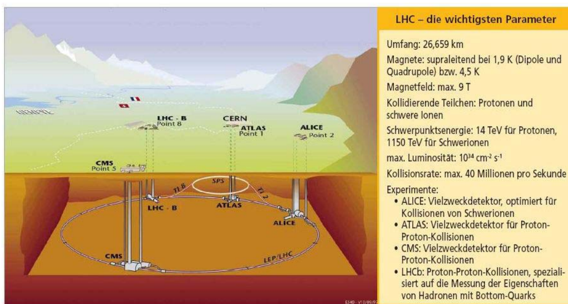
Abbildung 3: Skizze des LHC-Tunnels am CERN (Quelle: KET 2002, S. 31).
