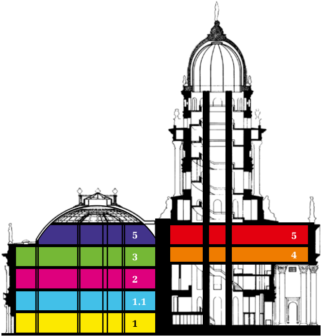
Schnitt durch den Deutschen Dom.
